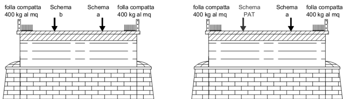
Figura 4.8 Esempio ricostruzione dello schema di carico previsto dalla normativa dell'epoca e sostituzione del carico principale con quello P.A.T. (esempio generico tratto dalla relazione di calcolo del ponte ad arco sul Rio Cavallo sulla SS 12 km 362.164, allegato BMS All.P3.2, normativa di riferimento Normale n.8 DEL 15/09/1933 M.LL.PP.) in condizione di traffico libero.
