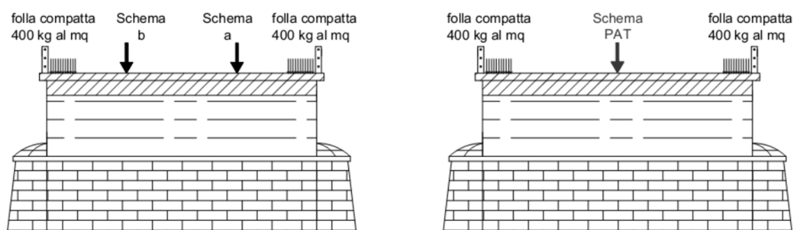
Figura 4.9 Esempio di sostituzione dei carichi con il carico PAT (esempio generico tratto dalla relazione di calcolo del ponte ad arco sul Rio Cavallo sulla SS 12 km 362.164, allegato BMS All.P3.2, normativa di riferimento Normale n.8 DEL 15/09/1933 M.LL.PP.) in condizione di transito del carico eccezionale in centro carreggiata e in assenza di spartitraffico o di altri dispositivi di ritenuta.
