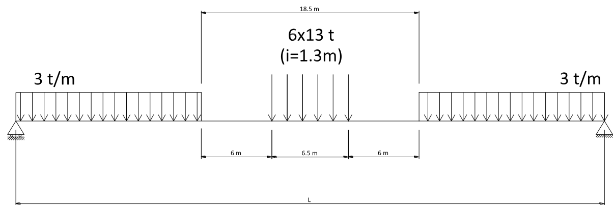
Figura 4.4 Schema di carico 6 assi x 13 t (interasse = 1.3 m) = 78 t
