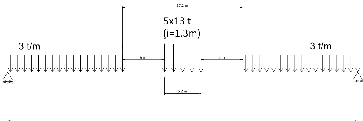
Figura 4.2 Schema di carico 5 assi x 13 t (interasse = 1.3 m) = 65 t
