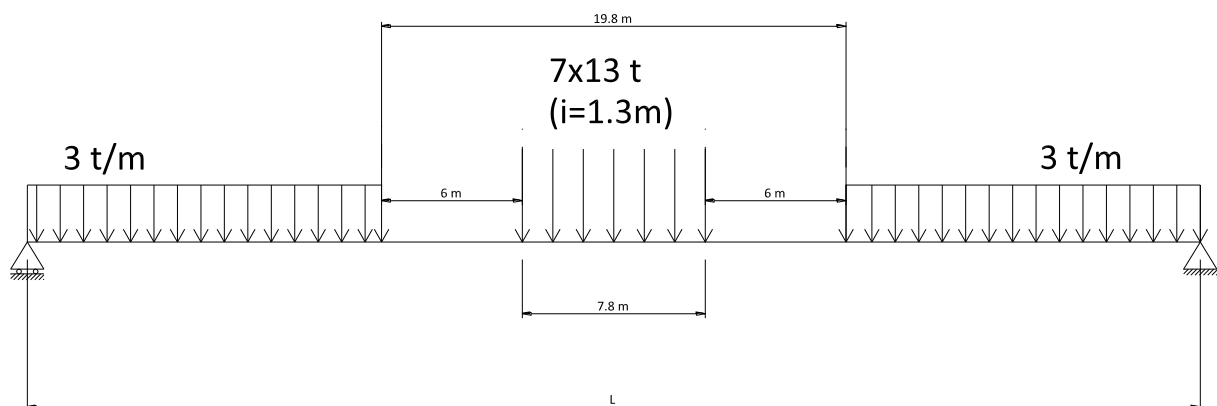
Figura 4.5 Schema di carico 7 assi x 13 t (interasse = 1.3 m) = 91 t
