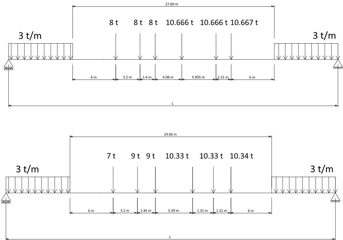
Figura 4.1 Schema di carico 56 t
